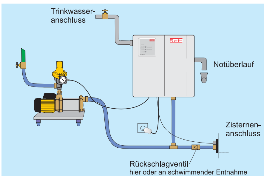
Installationsschema mit Aspri Hauswasserwerk
